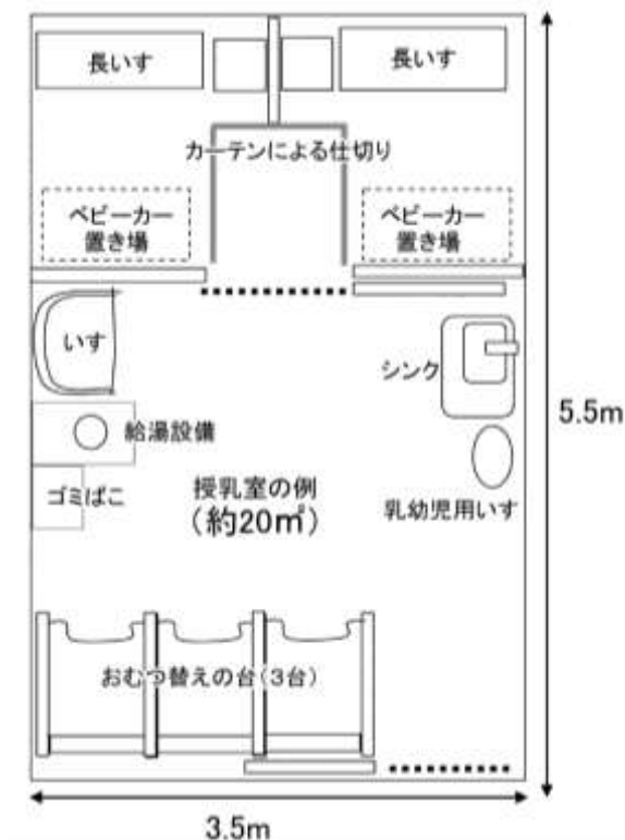
図 28 ベビーケアスペースの例 出典) 名古屋市福祉都市環境整備指針
