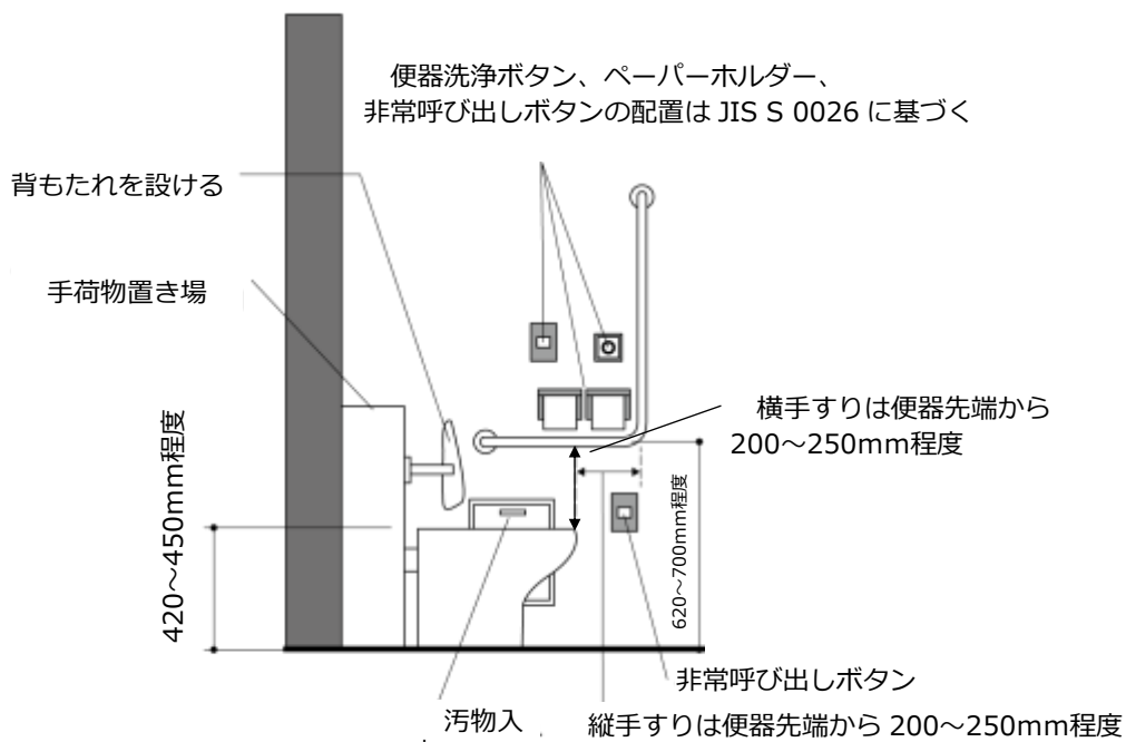
図25 便器周りの配置(例)
